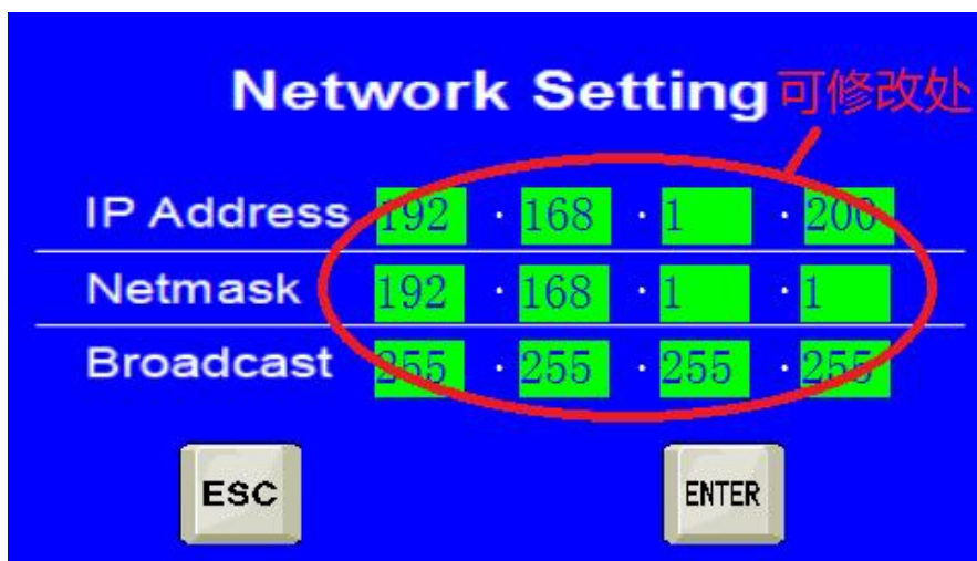
IP 查询/设置图
